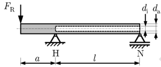
Modell mit Lagersteifigkeit
